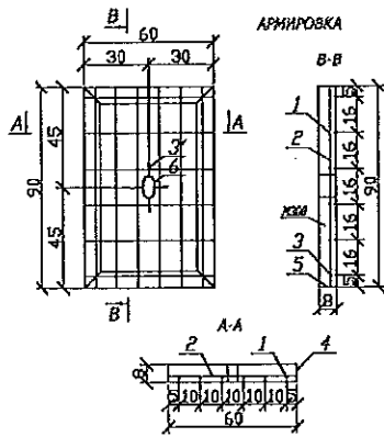
ДЕТАЙЛ НА КАПАК ЗА ШАХТА 60/90
