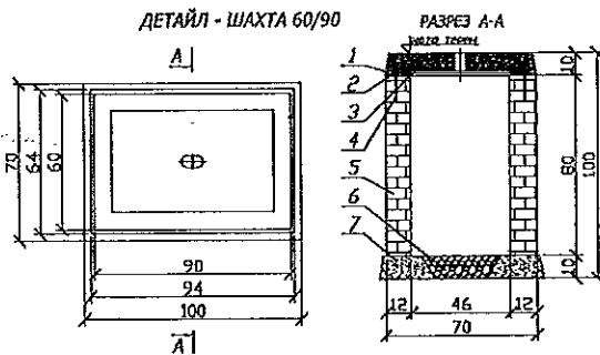
ДЕТАЙЛ - ШАХТА 60/90
